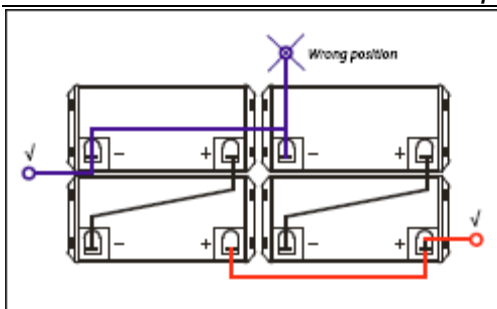
Wrong position – Nevhodné umístění Series-parallel connection – Sériově-paralelní zapojení
